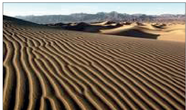
Abb 4: Diese Sanddünen entstanden durch Windverwehungen. Kalifornien, USA (AGI ha469y © Marli Miller, University of Oregon)
