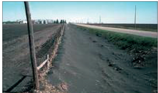
Abb 3: Verwehter Oberboden wurde in einem Straßengraben abgelagert. Iowa, USA (AGI hkeamf © NRCS)
